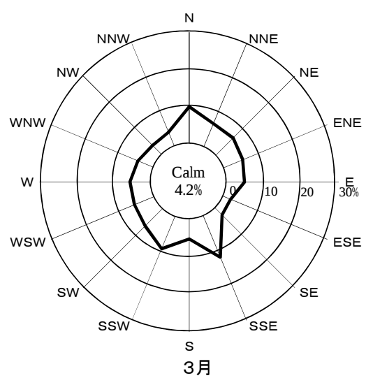
図Ⅲ.2.1(2) 大阪府熊取オフサイトセンター局風配図
